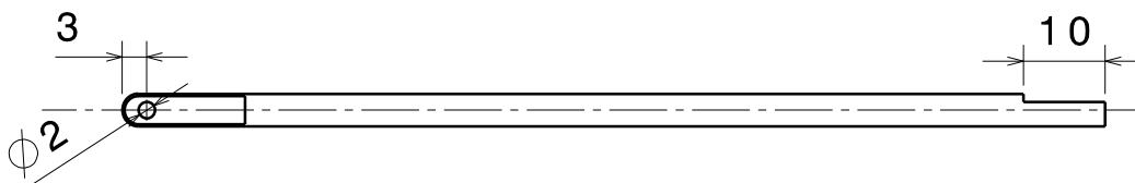
Vorderansicht Maßstab: 1:1
